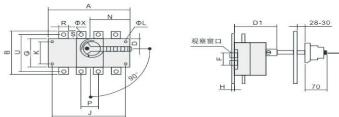
BRHGL-160~630/3(4)J柜外操作, 外形尺寸及安装尺寸
