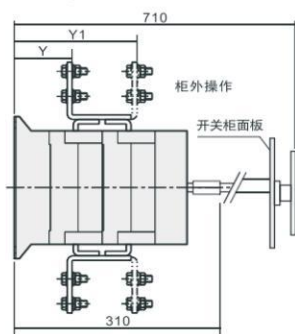
BRHGL-2000~3200/3 (4) J 柜外操作，外形尺寸及安装尺寸
