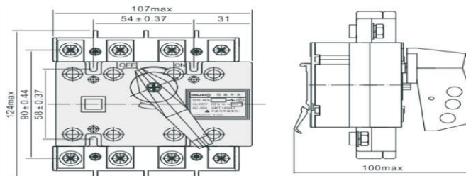
BRHGL-100/3(4) 隔离开关的外形尺寸及安装尺寸
