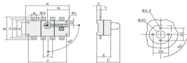
BRHGL-160~630/3(4)柜内操作, 外形尺寸及安装尺寸 柜外手柄安装尺寸
