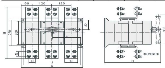
BRHGL-2000~3200/3(4) 柜内操作, 外形尺寸及安装尺寸
