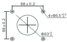
A 型柜外手柄座安装尺寸
