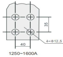
BRHGL-800~1600/3(4)柜内操作, 外形尺寸及安装尺寸
