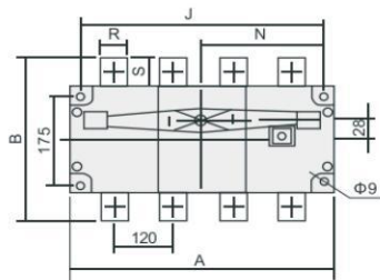
BRHGL-800~1600/3(4)J柜外操作, 外形尺寸及安装尺寸
