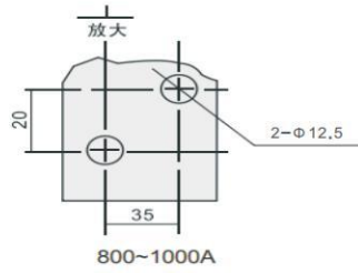
BRHGL-800~1600/3(4)柜内操作, 外形尺寸及安装尺寸
