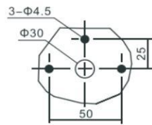
B 型柜外手柄座安装尺寸
