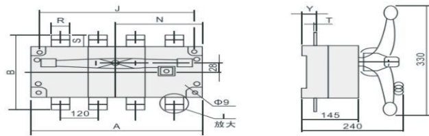
BRHGL-800~1600/3(4)柜内操作, 外形尺寸及安装尺寸
